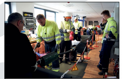
AUS-TEAMS FÜR ABZWEIGMUFFEN
